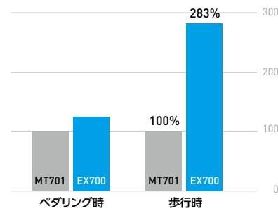
ペダリング時/歩行時におけるミッドソール変位量
