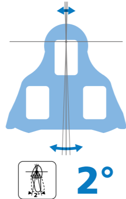
SM-SH12 フロントセンターピボッティングモード 回転の支点がフロントで左右に少し遊びがあります カラー: ブルー
